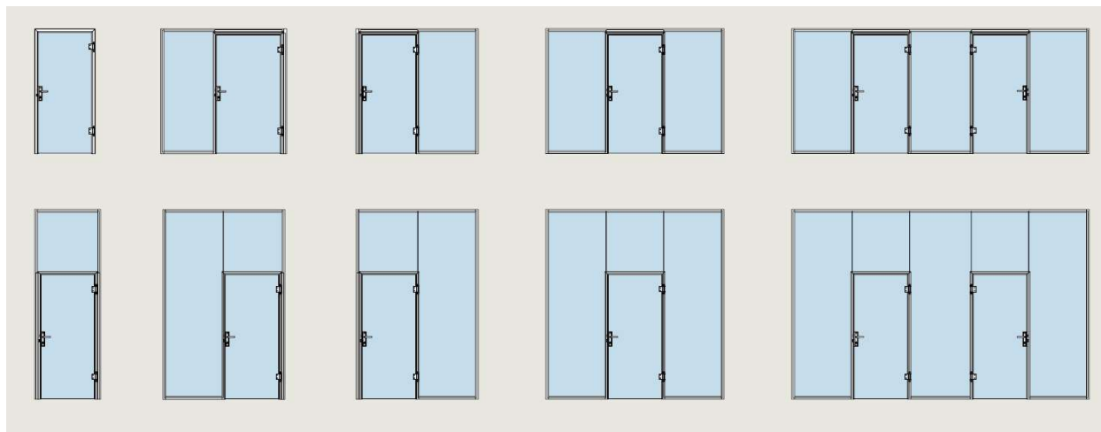
Šema izvođenja pregrada sa staklenim vratima
