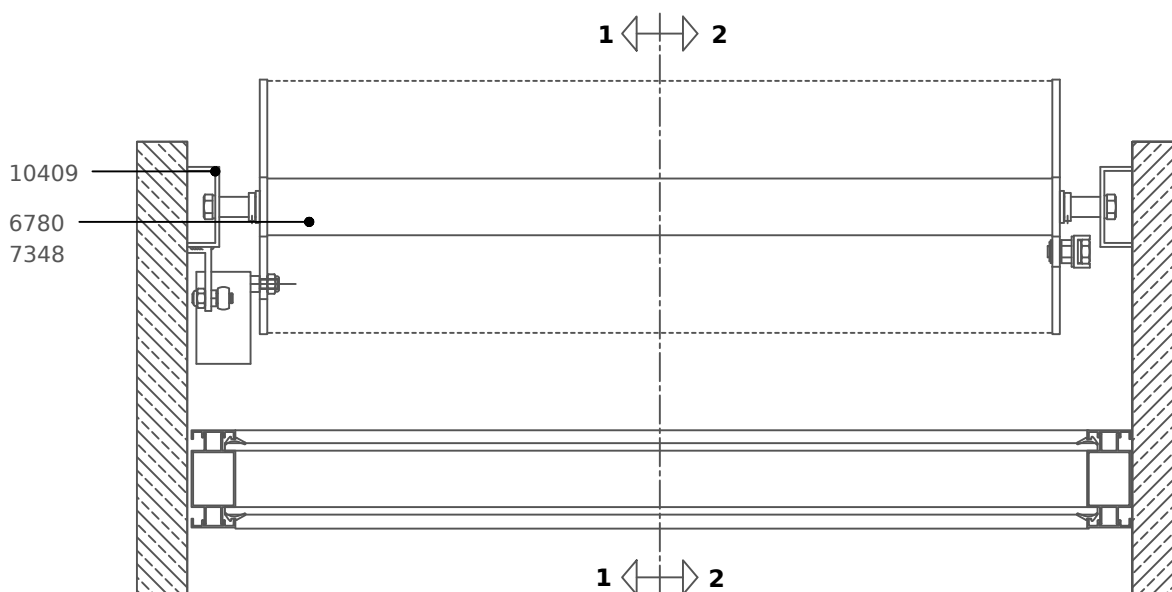
PRESEK A-A
