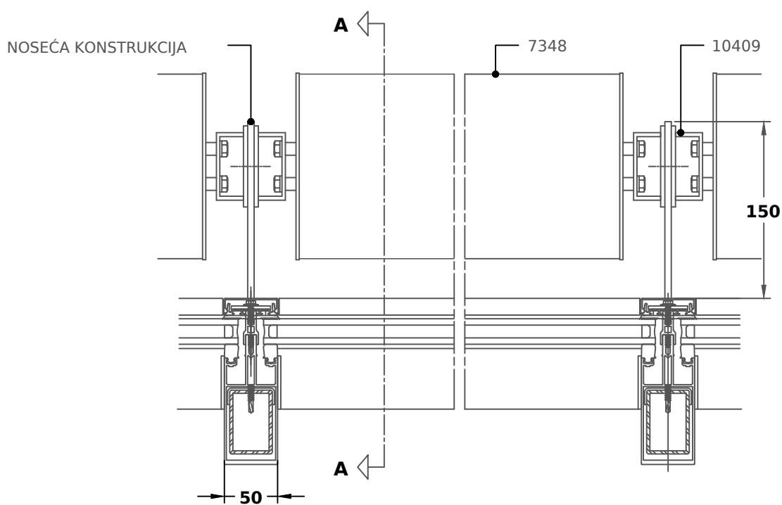
PLAN Razmera 1:5
