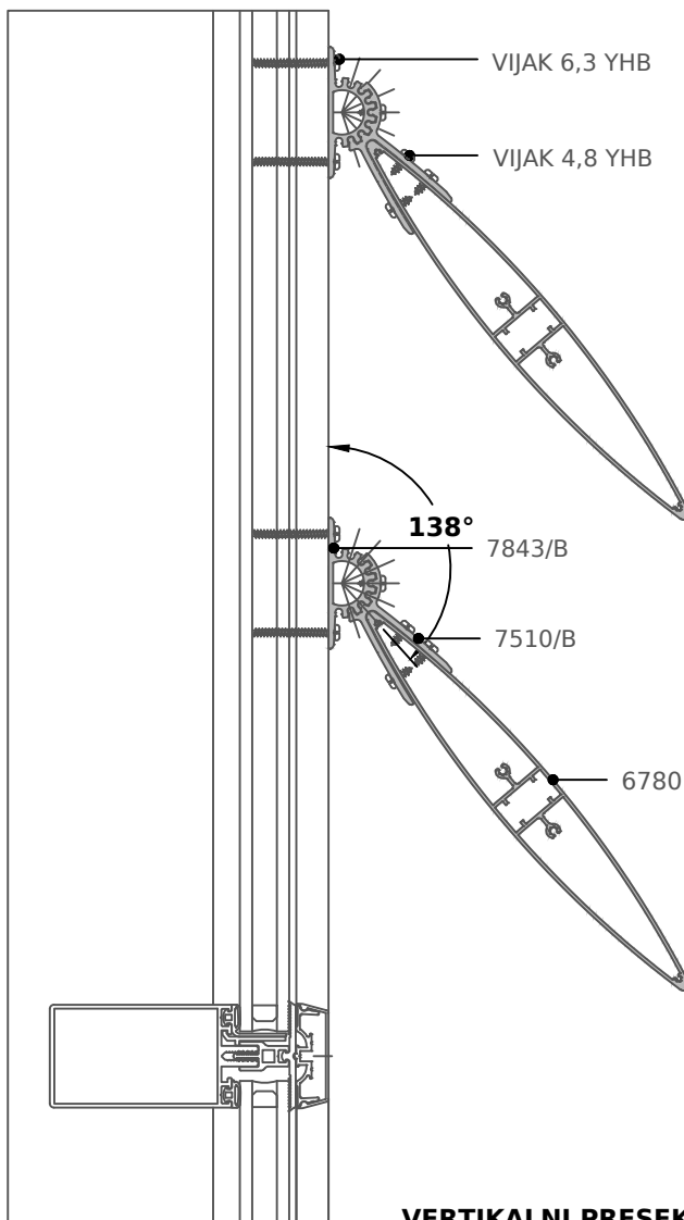
VERTIKALNI PRESEK
