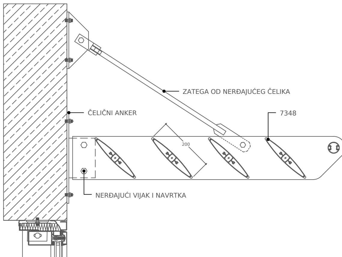
PRESEK A-A
