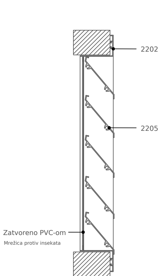
PRESEK A-A
