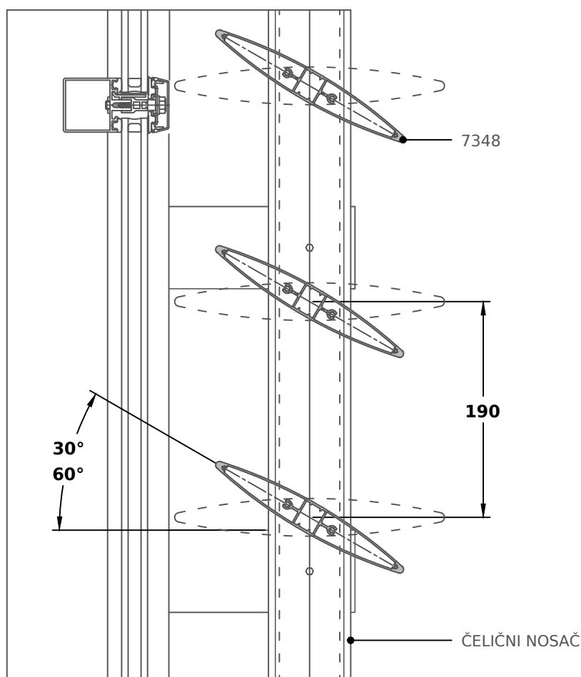
PRESEK A-A
