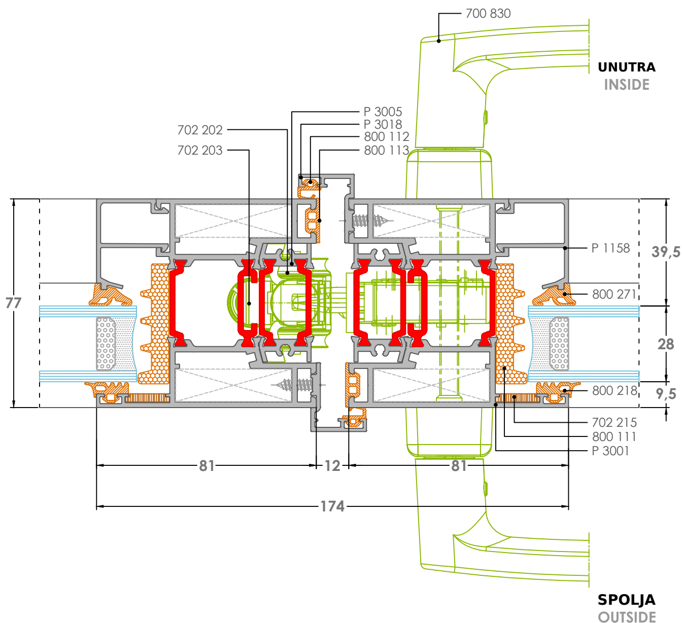
11K DETALJ-Detail
