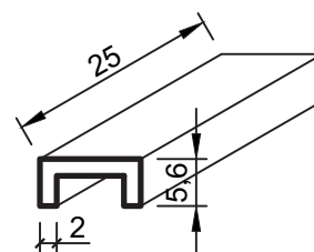
No : 295 ( Mera rezanja 50 mm ) 0,110 kg/m
