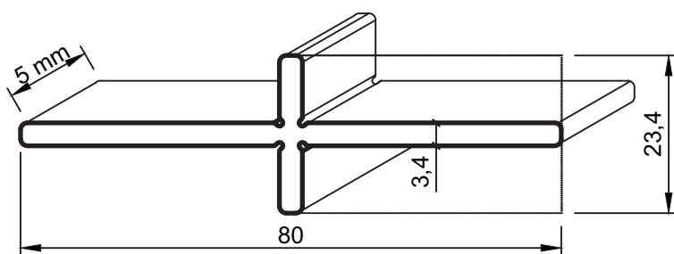
No : 286 Distancer 5 mm 0,900 kg/m
