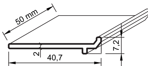
No : 244/B Naslon stakla ( Mera rezanja 50 mm ) 0,250 kg/m
