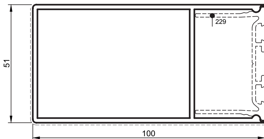
NO : 228 Poklopac (100 mm) 1,600 kg/m
