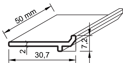
No : 244 Naslon stakla ( Mera rezanja 50 mm ) 0,190 kg/m
