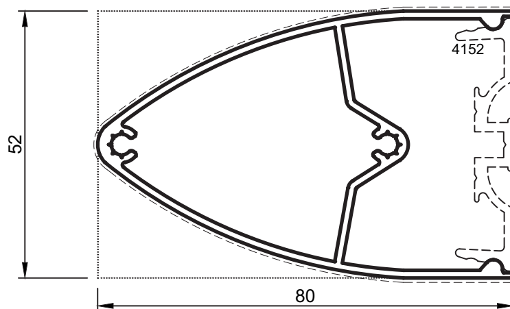
NO : 283 Badem Poklopac 1,045 kg/m
