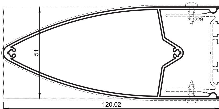
NO : 6370 Manji badem Poklopac 1,280 kg/m
