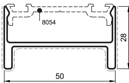
NO : 8068 28 mm Poklopac 0,560 kg/m
