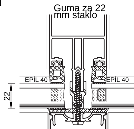
VERTIKALNA DETALJI MULLION DETAIL
