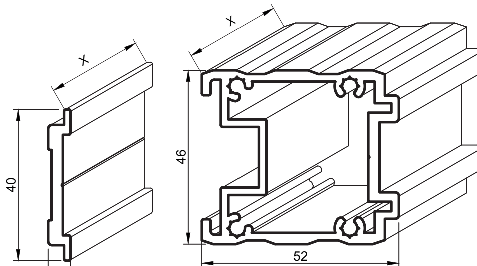
No : 239 Nosač spojnice 0,360 kg/m
