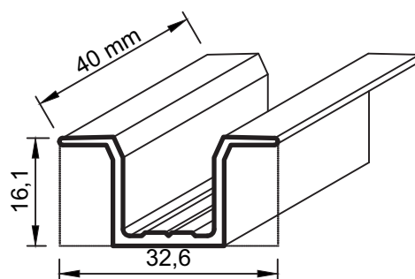
No : 199 Držać stakla ( Mera rezanja 40 mm )
