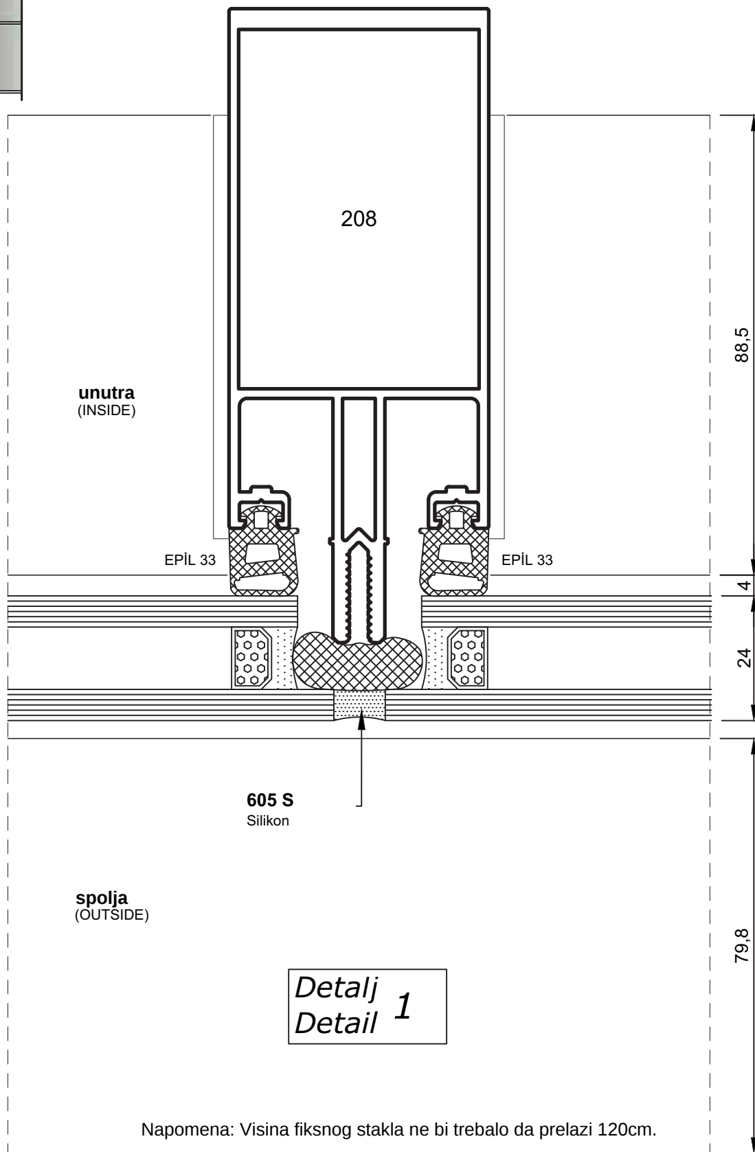
Detalj vertikalnog zastakljivanja STRUCTURAL GLAZING VERTICAL DETAIL
