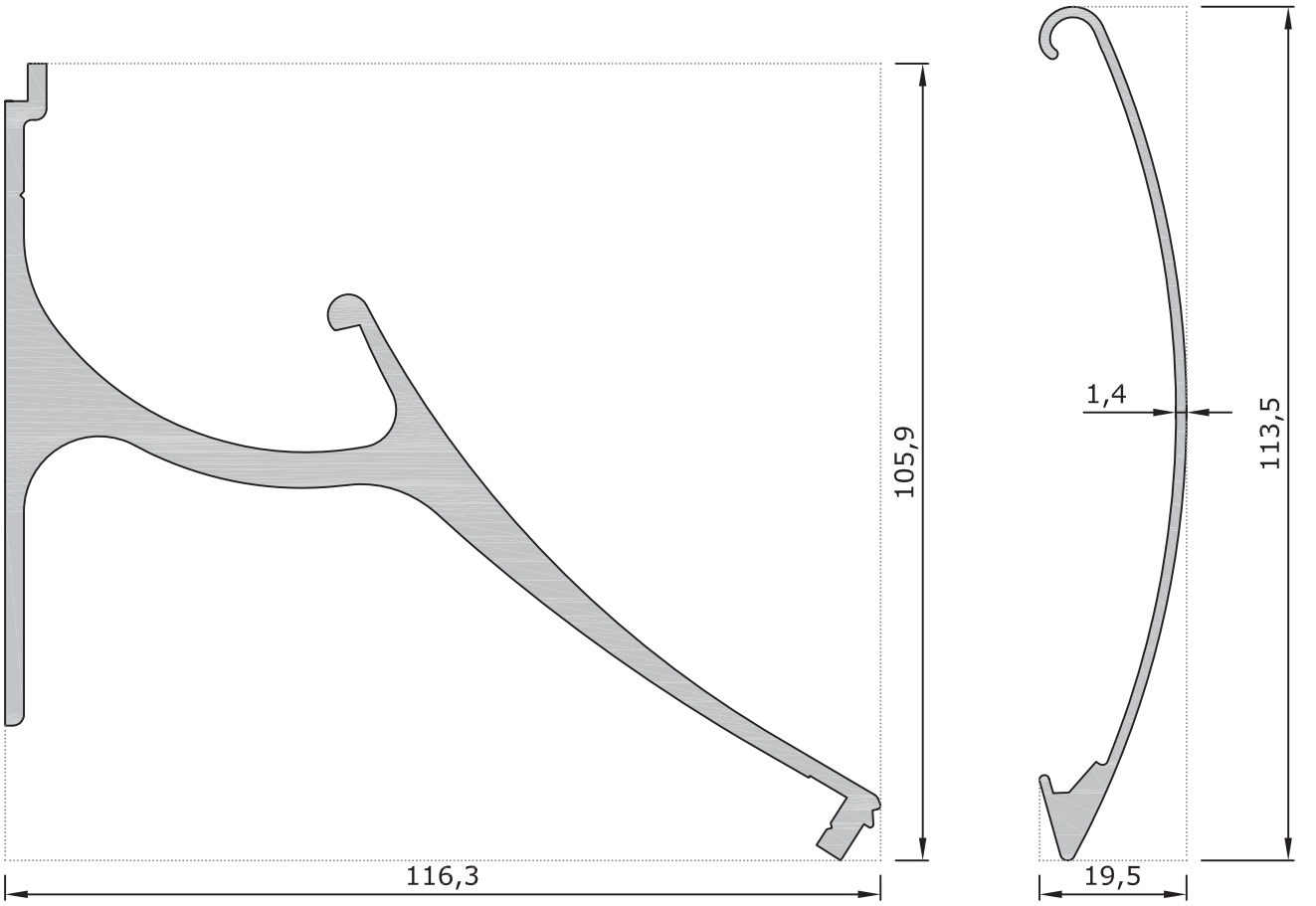
10419 | Güneş Kırıcı Montaj Pr. 2,845 kg/m | Connector Profile
