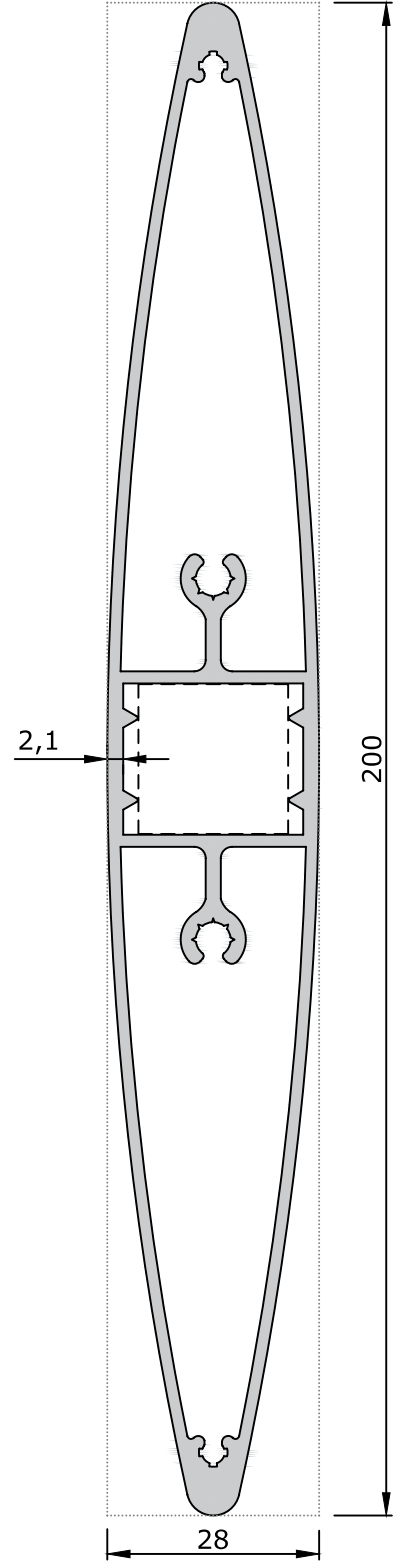
7348 | 200 mm Güneş Kırıcı Pr. 2,515 kg/m | 200 mm Sun Breaking Profile
