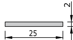
*9600 | 25X2 mm Lama Kılavuz Pr. 0,140 kg/m | Guide Profile
