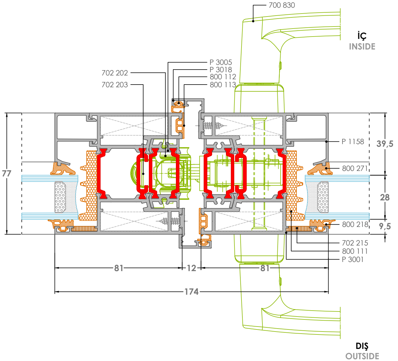
11K Detay-Detail
